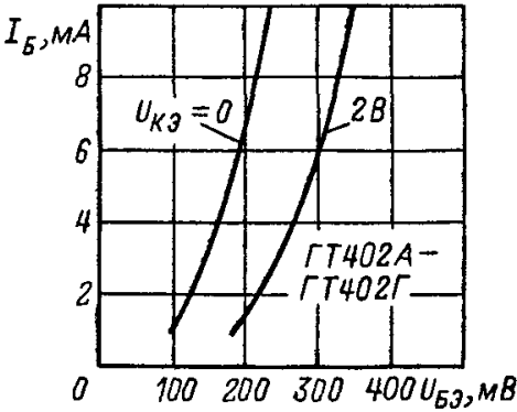
Входные характеристики
