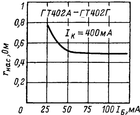
Зависимость сопротивления насыщения от тока базы.
