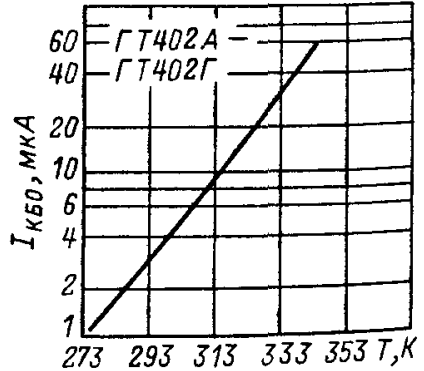
Зависимость обратного тока коллектора от температуры.
