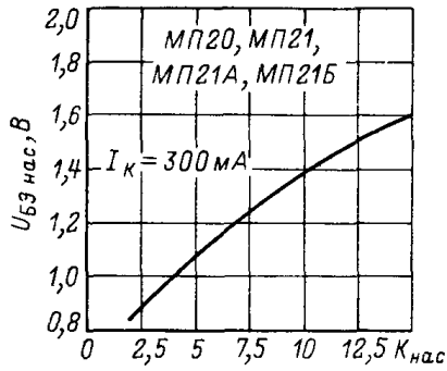
Зависимость напряжения насыщения база-эмиттер от коэффициента насыщения
