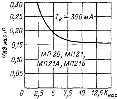
Зависимость напряжения насыщения коллектор-эмиттер от коэффициента насыщения
